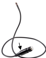
Abb. 6: Sonde Wöhler VE 400, Ø 5,5mm, Taste zum Umschalten der Blickrichtung mit Pfeil markiert.
